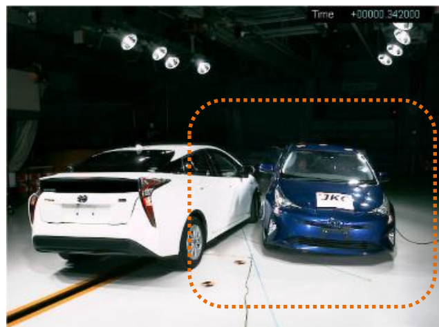
0.34 秒 (340ms) 後にローリング角は左に 5.4°
