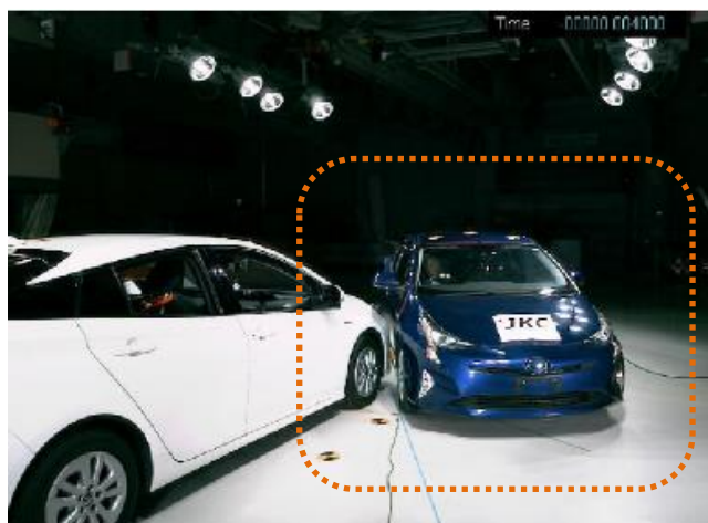
0 秒 (0ms) 衝突開始
