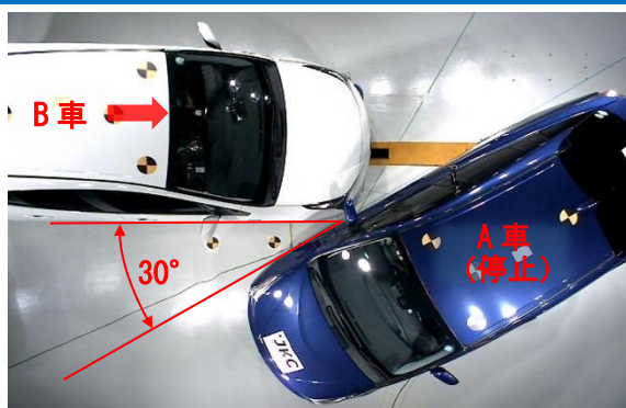
写真 1（衝突速度 25km/h 衝突角度：30°）
