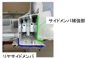
リヤサイドメンバ、サイドメンバ補強部カット断面
