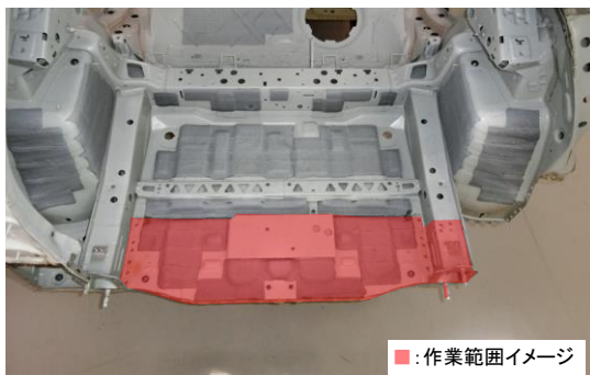
トランクルームフロア後部、リヤサイドメンバ後部、サイドメンバ補強部後部取外し状態
