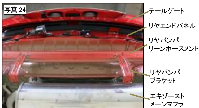
下面視
