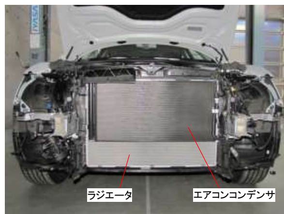
サイドリインホースメント取外し状態
