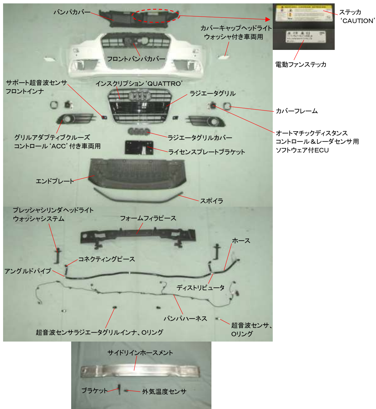
フロントバンパカバー、サイドリインホースメント
