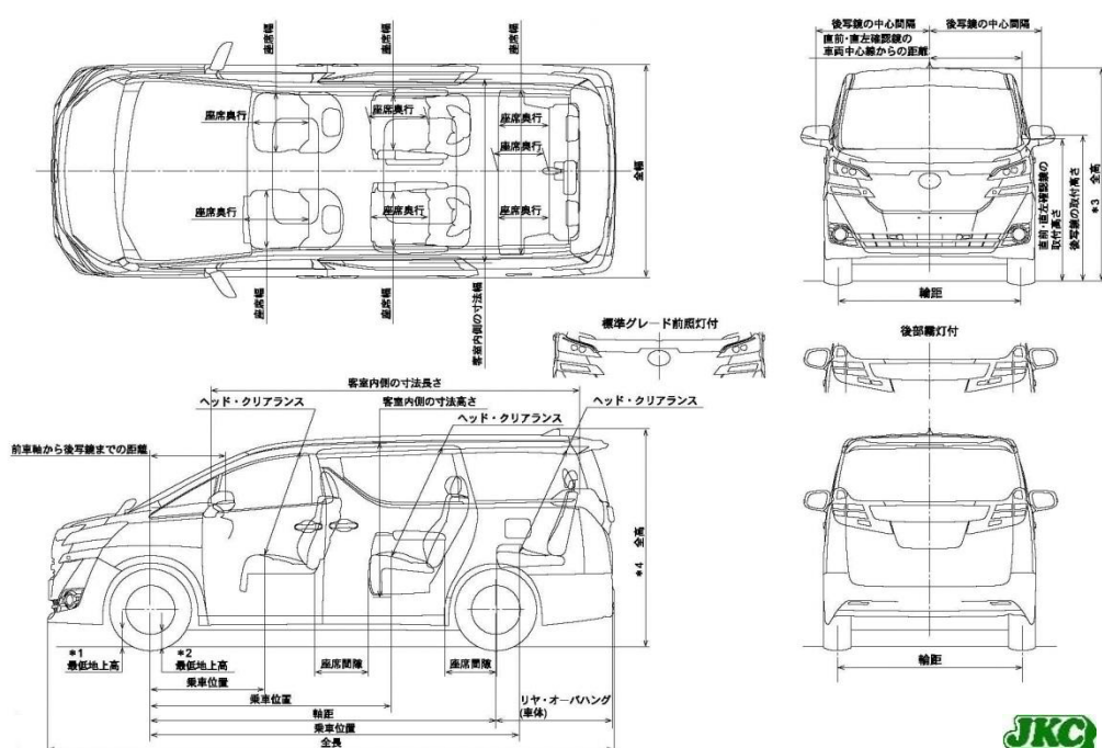
四面図
