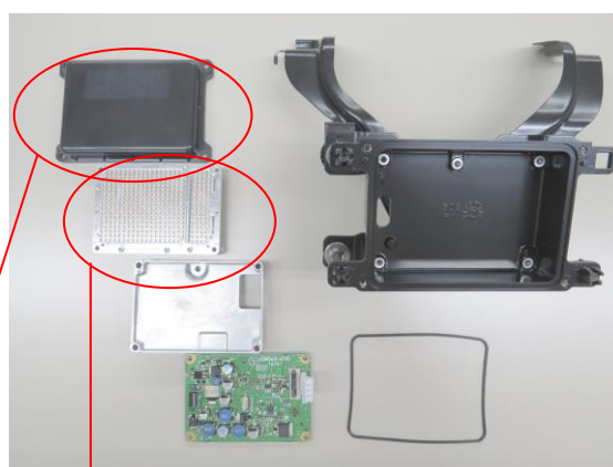
写真5 ミリ波レーダ例
