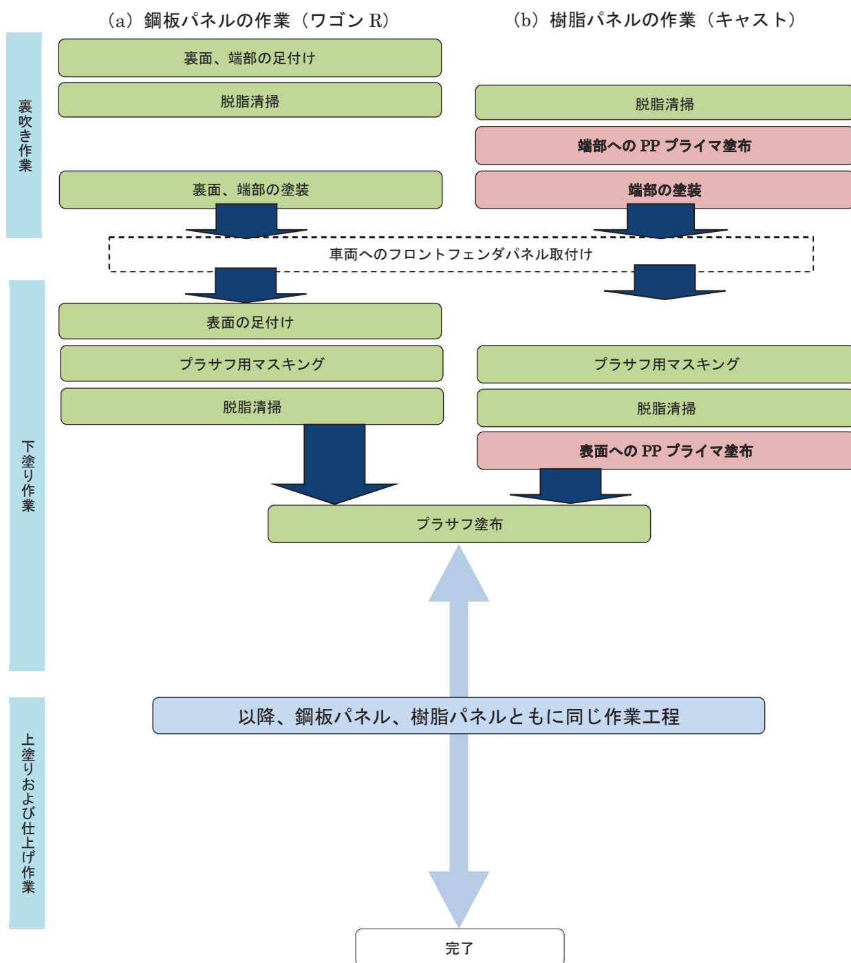
図 1. 鋼板パネルと樹脂パネルの補修塗装作業の比較（フロントフェンダパネル）
