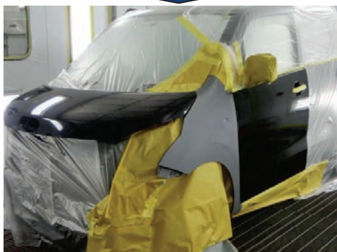
写真 14. 上塗りマスキングの状態
