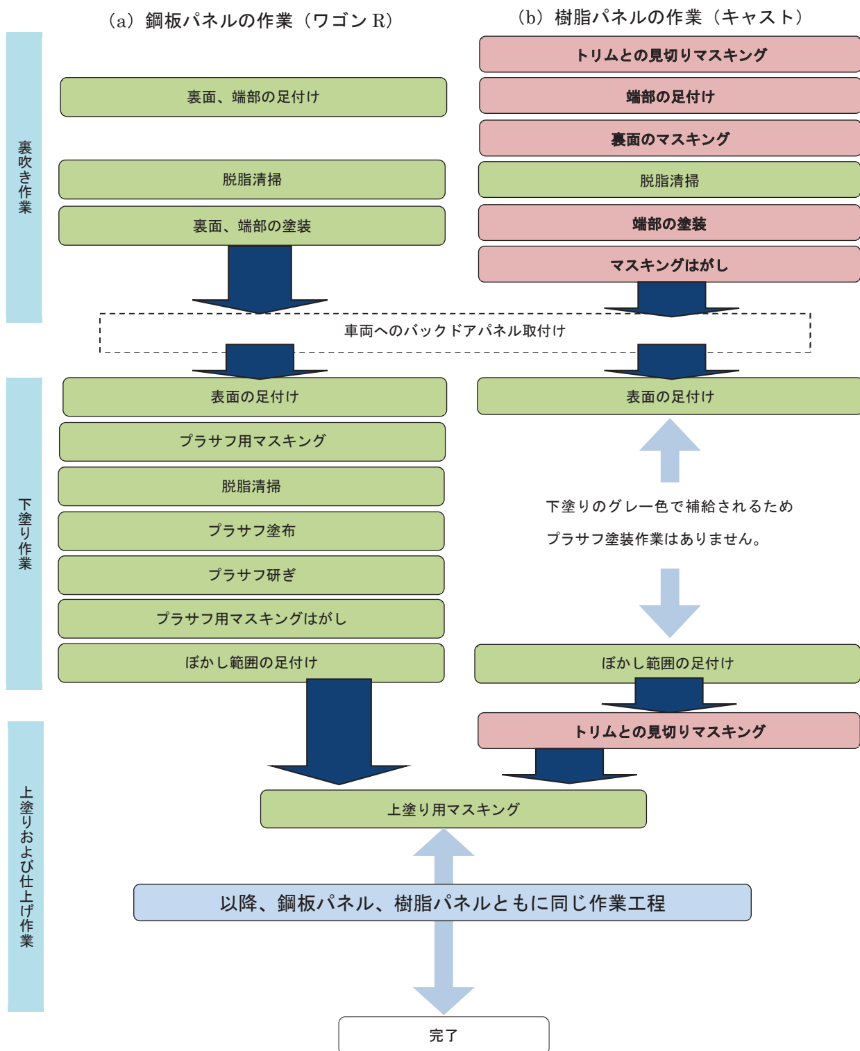
図 2. 鋼板パネルと樹脂パネルの補修塗装作業の比較（バックドアパネル）
