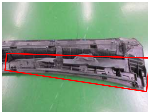
ベンチレータルーバ裏側補強（30 系）
