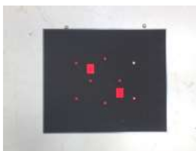
リフレクタ (レーザレーダセンサ光軸調整用)
