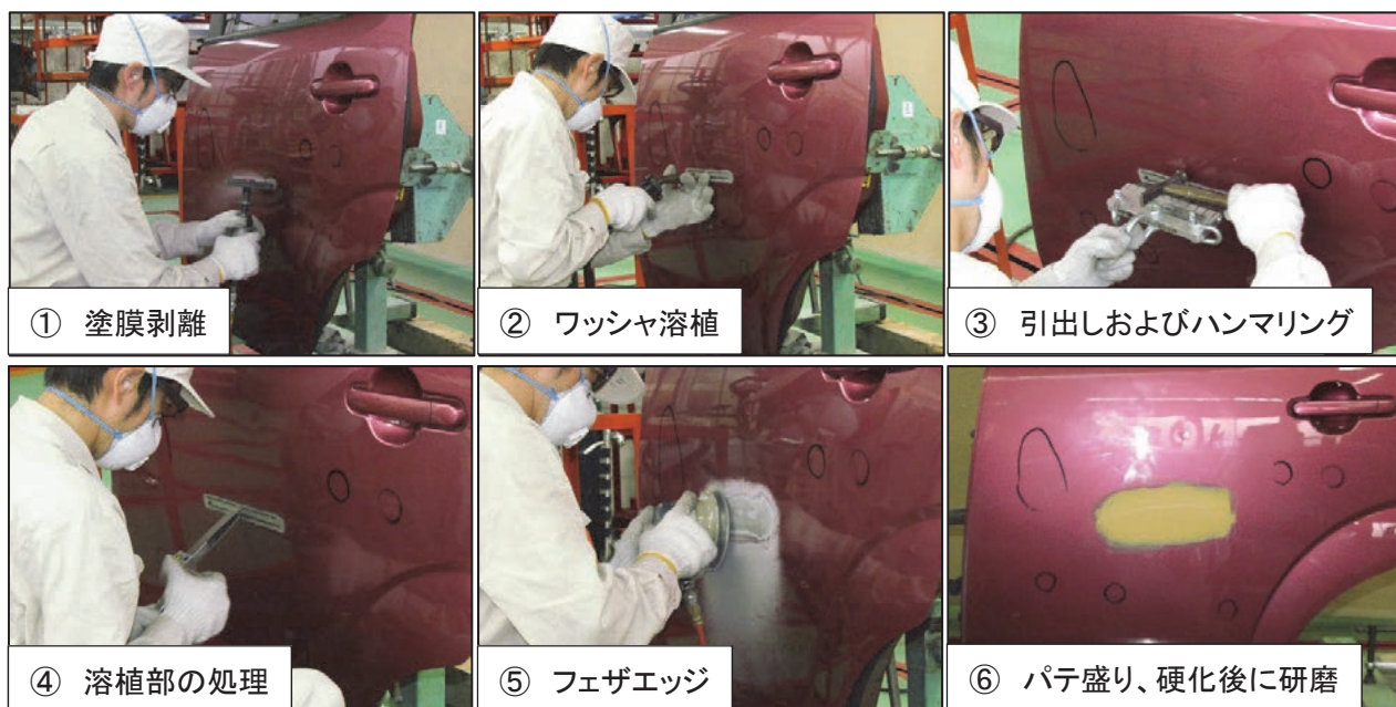
ワッシャ溶植機 SW-3700
