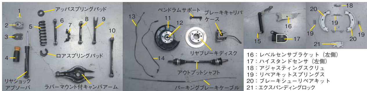
リヤサスペンション構成部品(片側)
