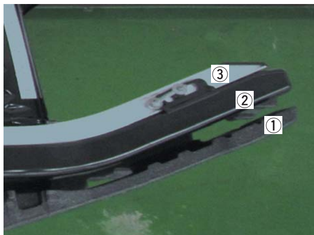
部品名称 ①フロントバンパエネルギーアブソーバ ②ポップアップフードチャンバ ③フロントバンパラインホースメント
