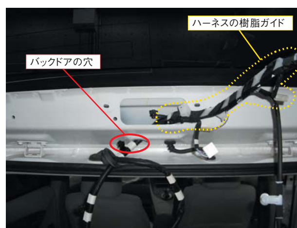
図4 バックドアハーネス貫通部
