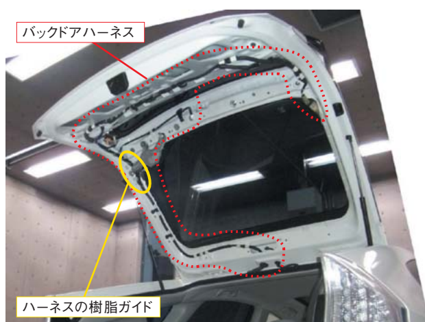
図3 バックドアハーネスの取付き状況
