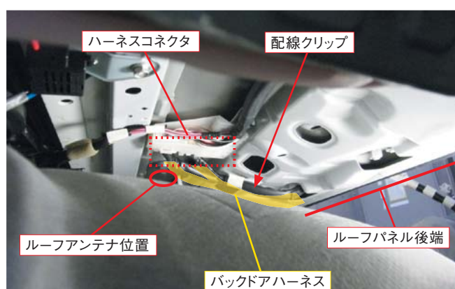
図5 車体側のハーネスコネクタ切り離し位置
