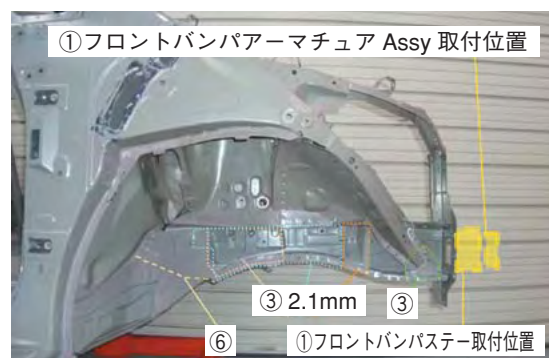
サイドフロントメンバ右外側
