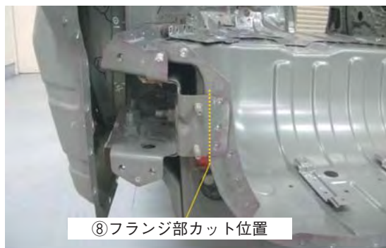
リヤ上側（リヤリヤフロア取外し状態）
