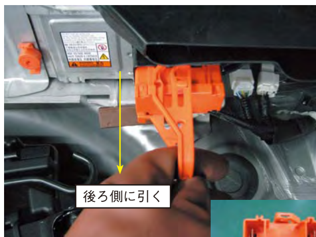
写真13 サービスプラググリップの取外し
