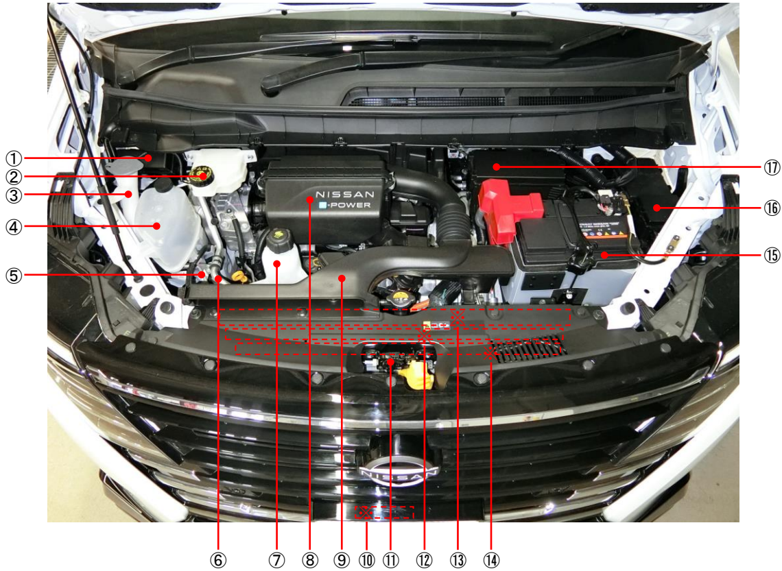
① HR14DDe(1, 433cc)直列3気筒DOHC(発電用)エンジン+EM57モータ
