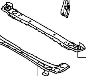
ラジエータロアフレームCOMP
