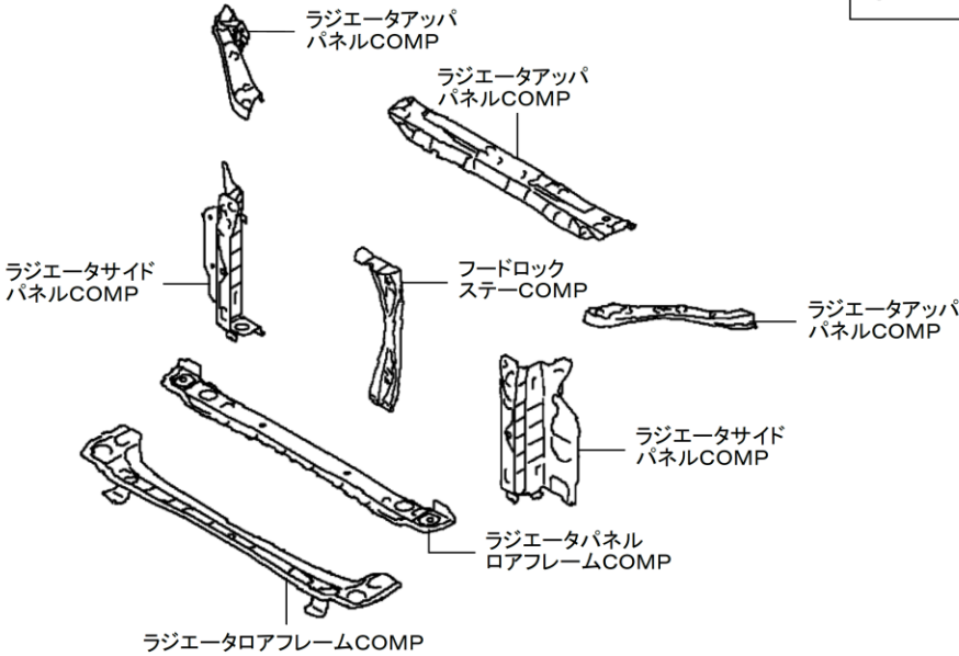
ラジエータロアフレームCOMP
