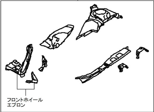
ホイールエプロンサブCOMP
