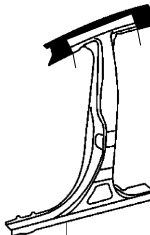
リヤボデーフロントアウトサイドパネル
