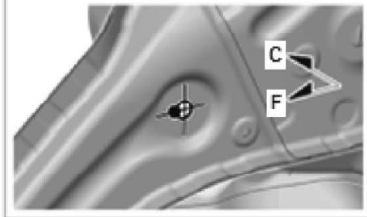
D3, d3 フロント・ホイールハウス アップ メンバ 基準穴 \phi 20
