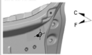
D4, d4 フロント・フェンダ後部上側 取付け穴φ9.0
