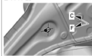
D3, d3 フロント・ホイールハウスアッパメンバ 基準穴φ20
