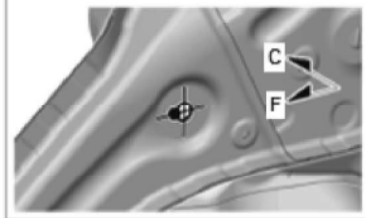
D3, d3 フロント・ホイールハウスアッパメンバ 基準穴 \phi 20
