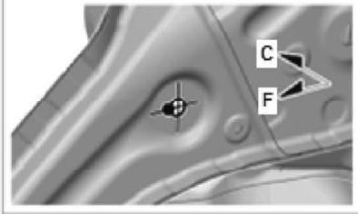
D3, d3 フロント・ホイールハウス アップル メンバ 基準穴 \phi 20
