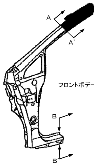
フロントボデーピラーラインホースメントサブAssyアッパ
