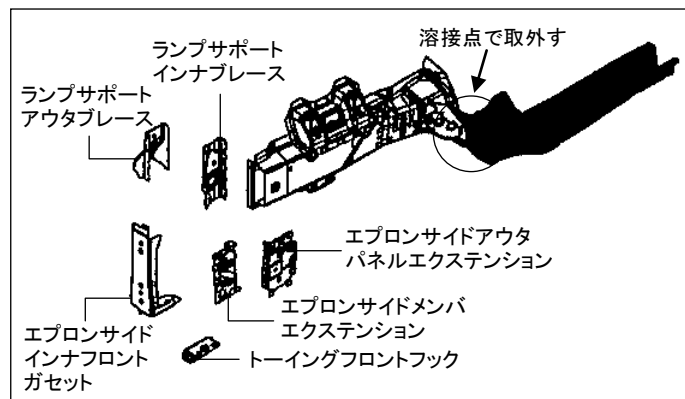
* フロントサイドメンバ
