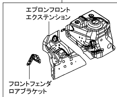
フェンダエプロンパネルセット
