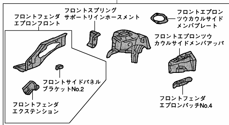
フロントフェンダエプロンAssy
